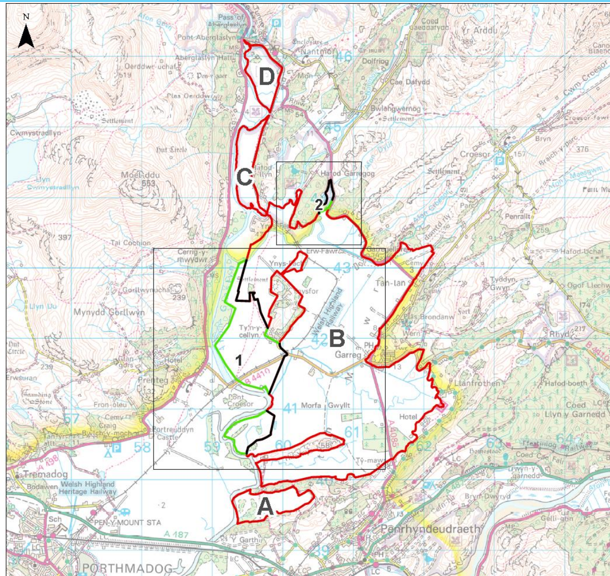
Ffigur 2. Ffiniau cyfredol ac arfaethedig ar gyfer ardal draenio mewnol Llanfrothen
